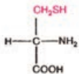
Цистеин (цис)
