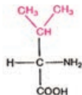
Валин (вал)
